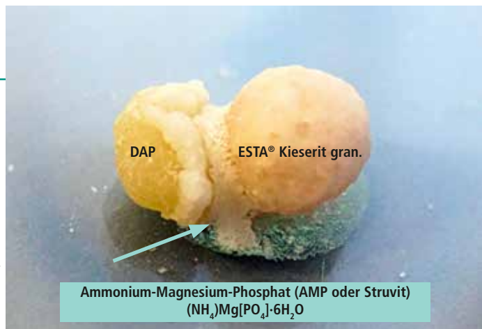
Abb. 1: Struvitbildung bei Kombination von DAP und ESTA® Kieserit gran. (im 1:1-Verhältnis unter Einfluss von Feuchtigkeit, diese Reaktion kommt so auch im Bodendüngerband zustande)
